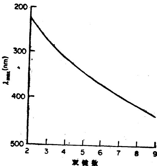
图 1.3 \alpha, \omega -二甲基多烯烃中最低能量跃迁的最大吸收波长
