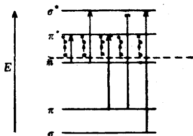
图 1.1 有机分子中各种可能的电子跃迁类型
