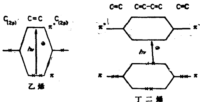
图 1.2 乙烯和丁二烯轨道能量
