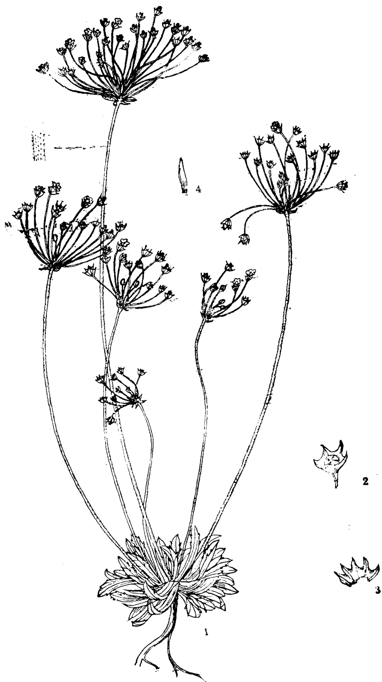
图版 3 1—4. 北点地梅 Androsace septentrionalis L. 1. 植株; 2. 蒴果和花萼; 3. 花萼展开; 4. 苞片。
