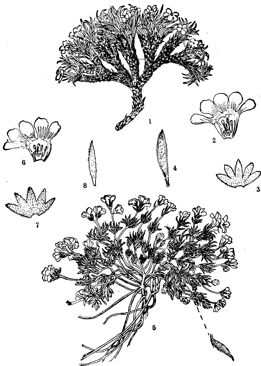
图版4 1—4.阿拉善点地梅 Androsace alashanica Maxim. 1. 植株; 2. 花冠展开; 3. 花萼展开; 4. 苞片。5—8. 白花点地梅 A. incana Lam. 5. 植株; 6. 花冠展开; 7. 花萼展开; 8. 苞片。
