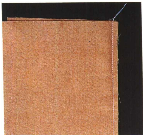
1. 两层布料反面相对叠合, 正面朝外, 布边对齐, 缉缝 0.4~0.5 厘米缝份。
