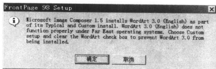
图 1-7 安装提示
