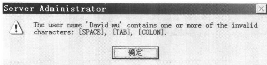
图 1-5 警告信息
