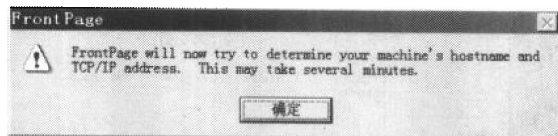
图 1-10 提示信息
