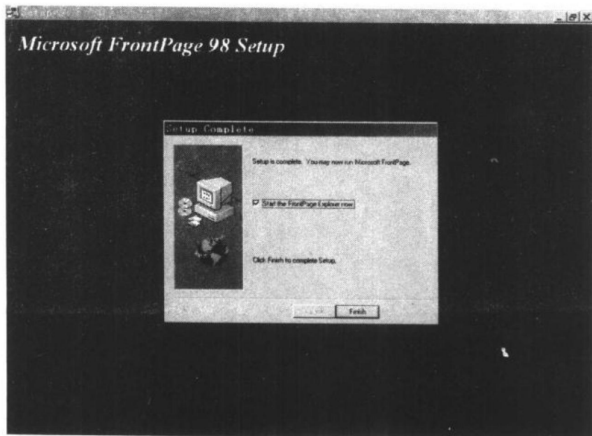
图 1-6 结束安装
