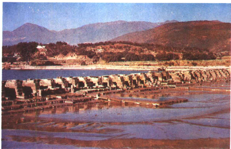
木兰陂
