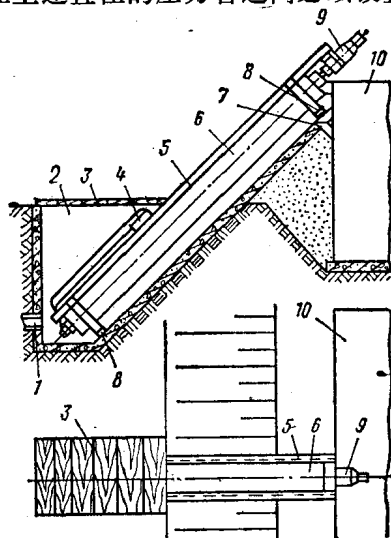
图1 螺旋泵装置示意
