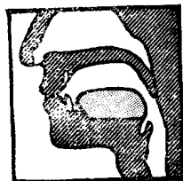
[p]
