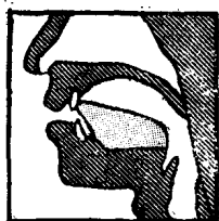
[t] [d]
