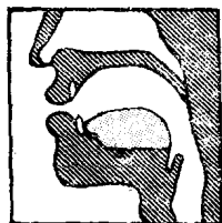
[ɛ]
