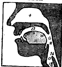
发音器官图
