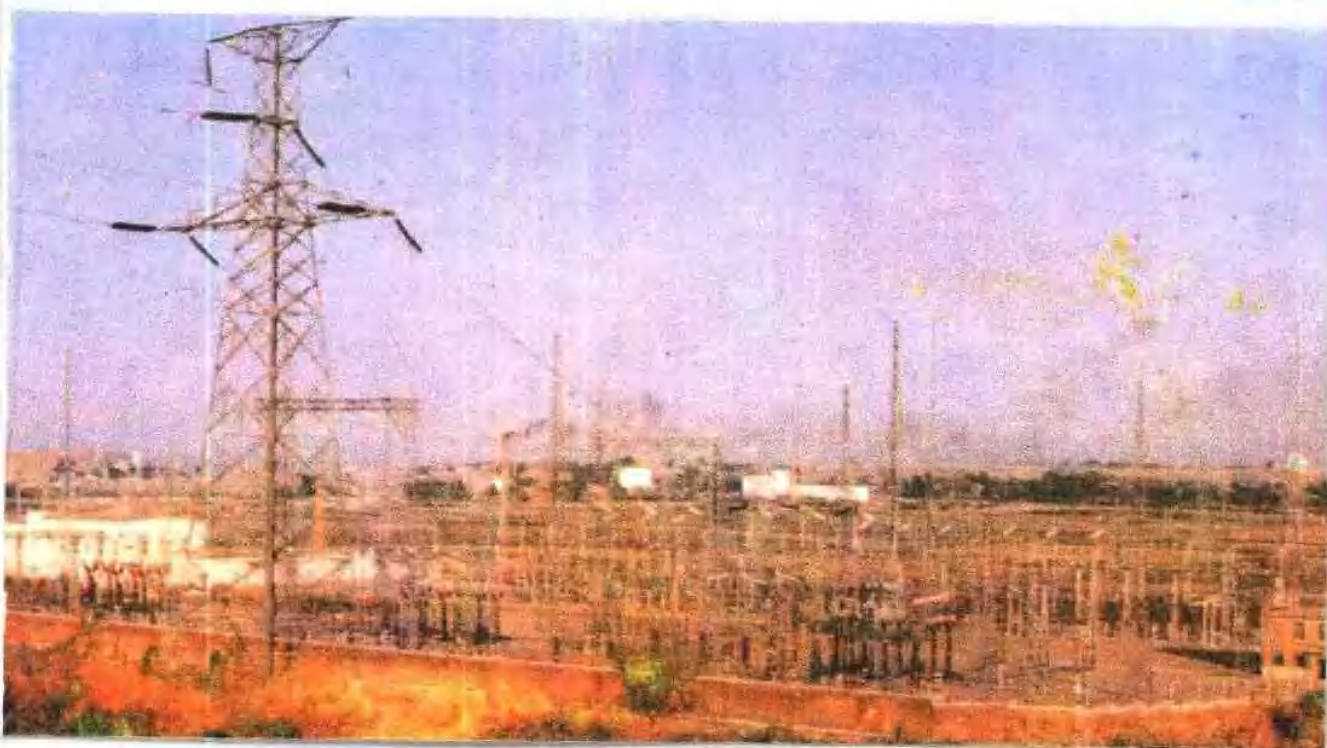
哈达湾一次变电所
