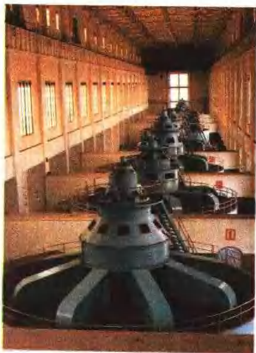
丰满发电厂 8 台水轮机组
