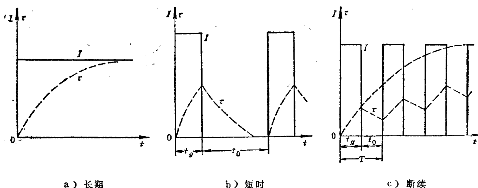
图37-1-3 电动机恒定负载运行状态示例
