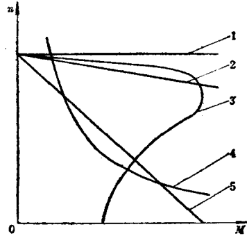
图37-1-2 电动机机械特性
