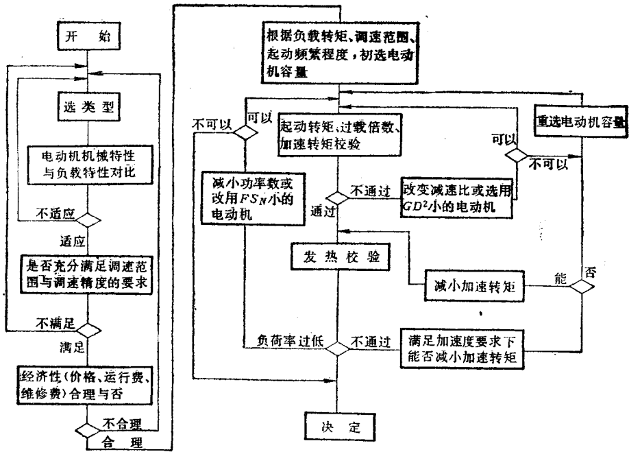
图37-1-1 电动机选择顺序
