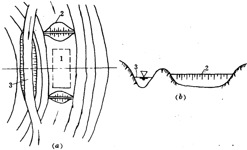
图 1 1 明渠导流示意图
