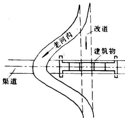
图 1-2 河槽改道示意图
