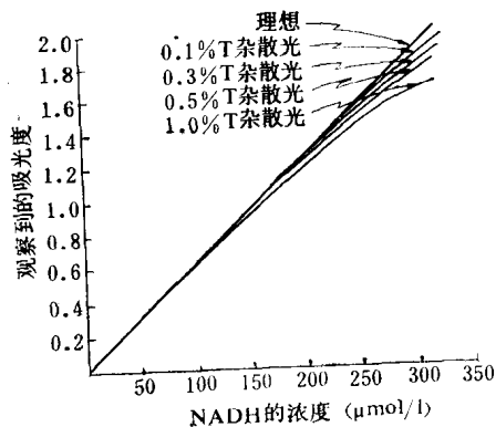
图1-4 杂散光对高浓度样品的影响
