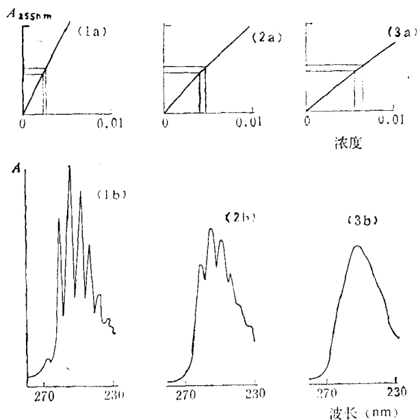
图1-2 狭缝宽度对吸收光谱和标准曲线的影响
