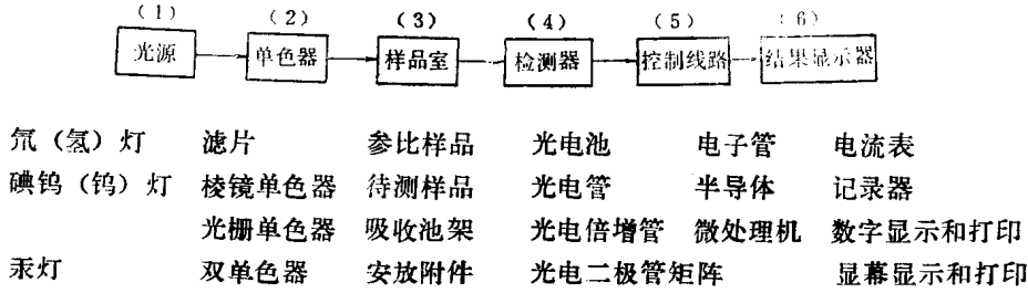
图1-5 紫外-可见-近红外分光光度计结构图
