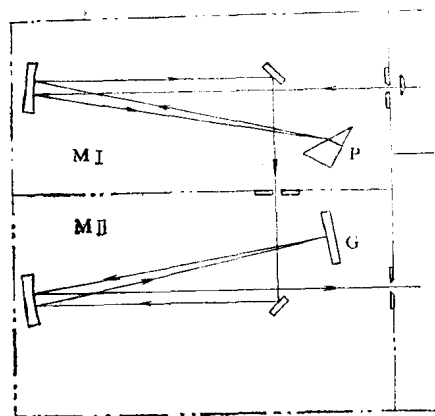
图1-8 双单色器MI和MII分别为第一和第二单色器
