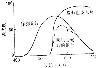
图1-6 滤光片的光谱特性
