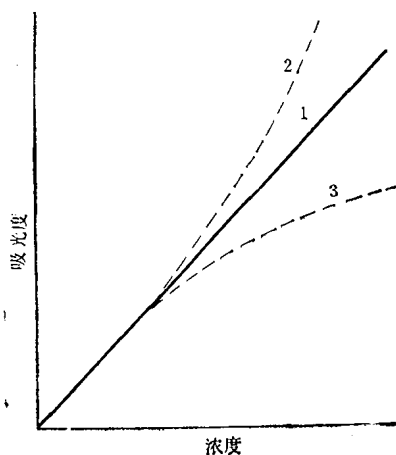
图1-1 比尔定律
