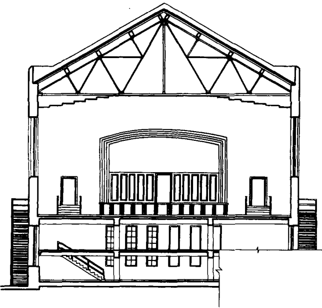
剖面 B-B
