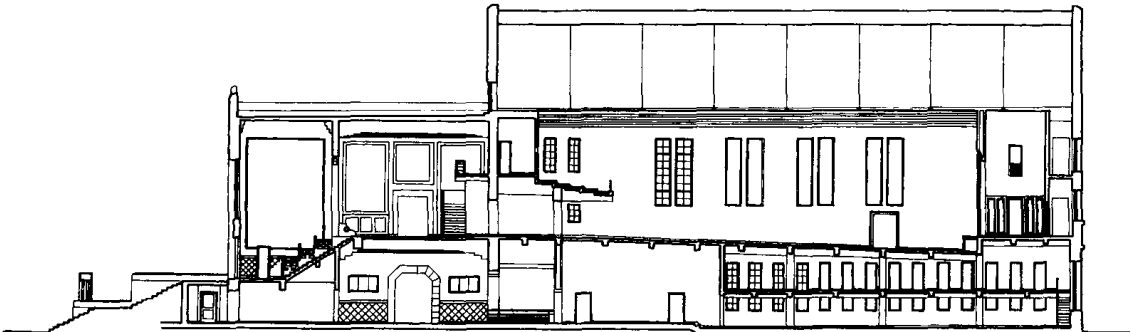
剖面 A-A
