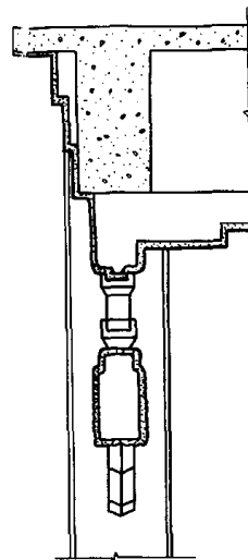
剖面
