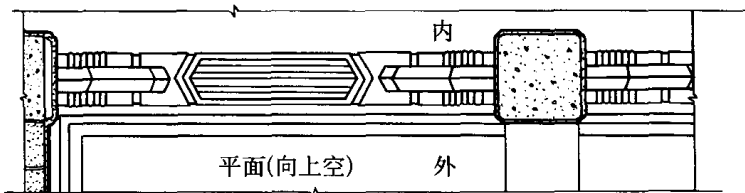
斗拱枋柱大样
