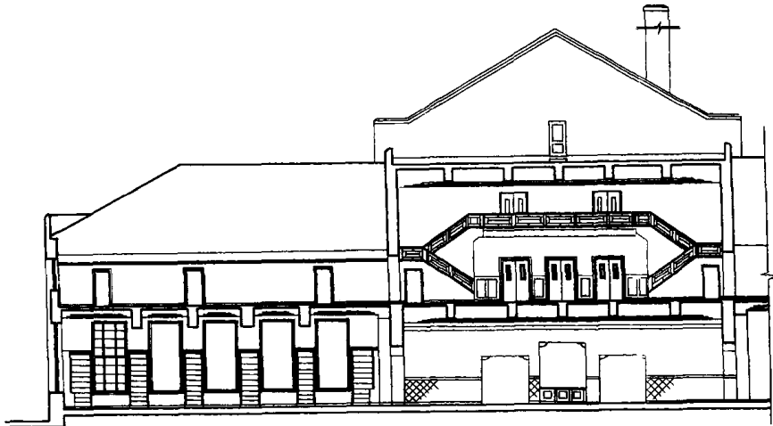
剖面 D-D
