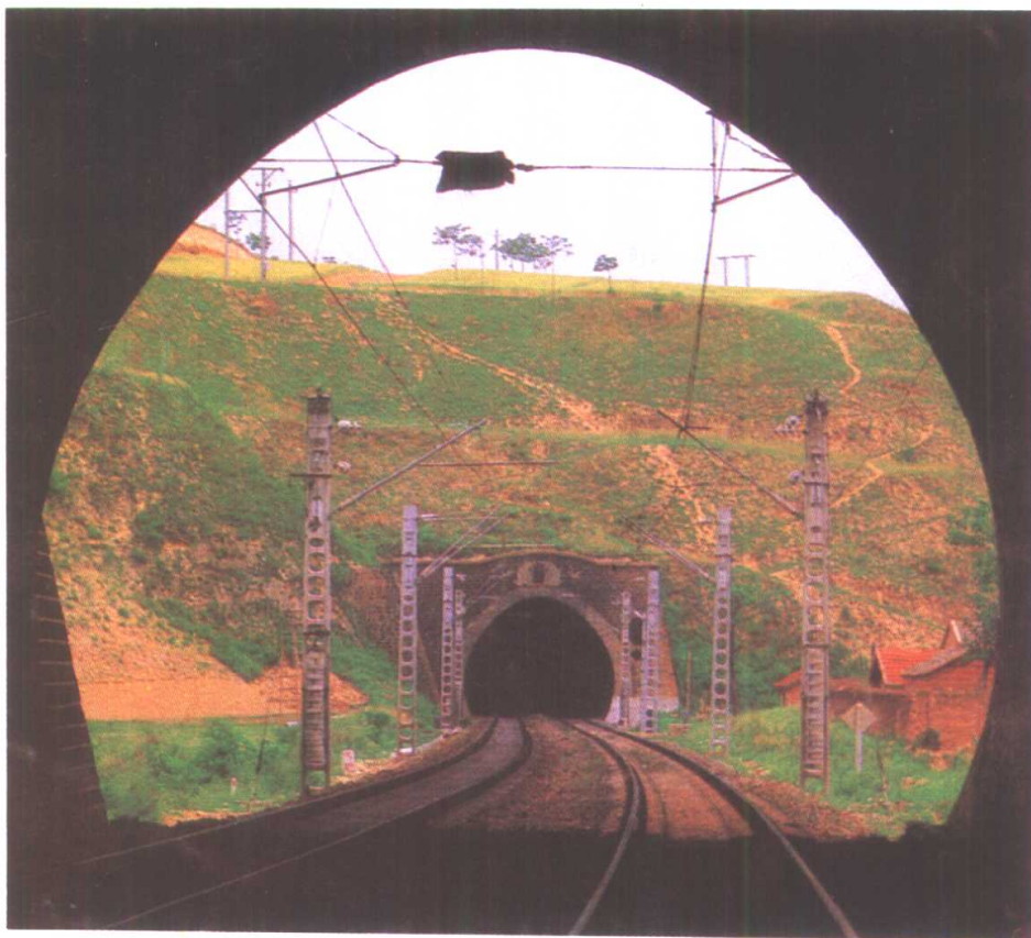
陇海线牛家庄双线隧道
