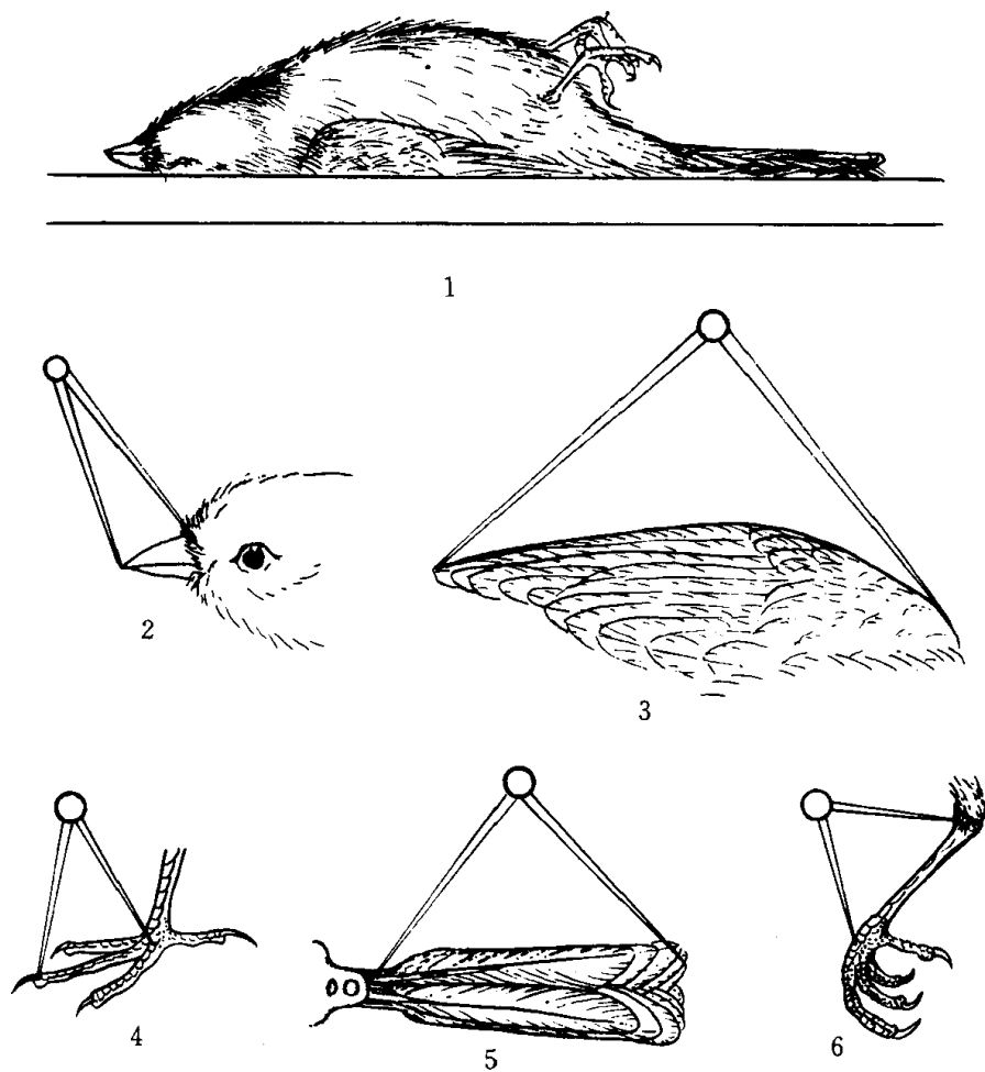
图2 鸟体测量法
