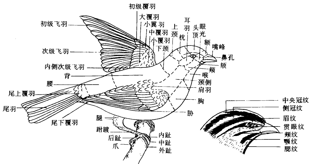
图 1 鸟体外形图
