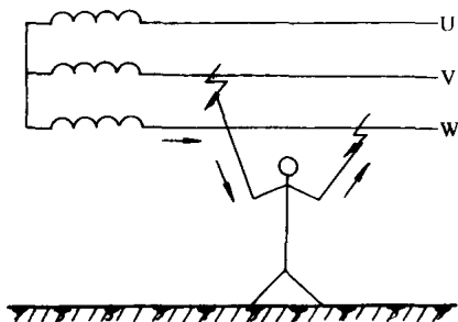
图 1-6 两相触电
