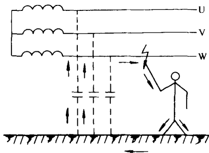
图 1-5 中性点不接地单相触电
