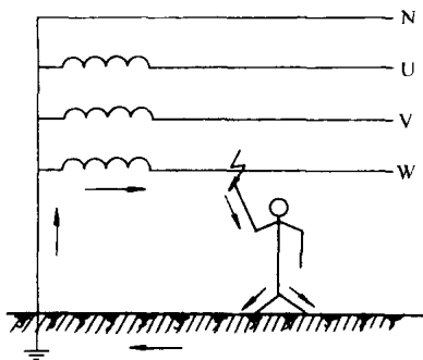
图 1-4 中性点直接接地单相触电
