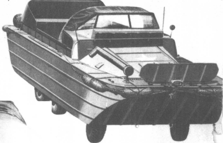
▲美国陆军“DUKW”(鸭子)式两栖 输送车。
