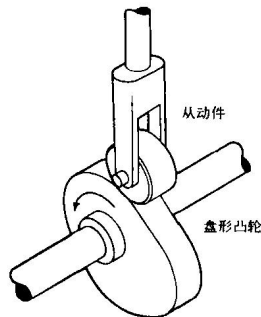
盘形凸轮及其从动件
