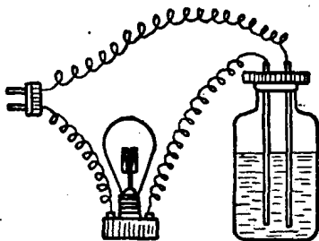
图12-1 试验物质导电性的装置
