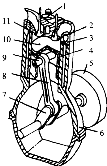
图1 四冲程柴油机构造示意图
