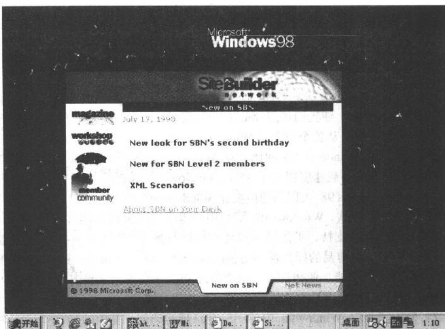
图 1-1-1 活动桌面
