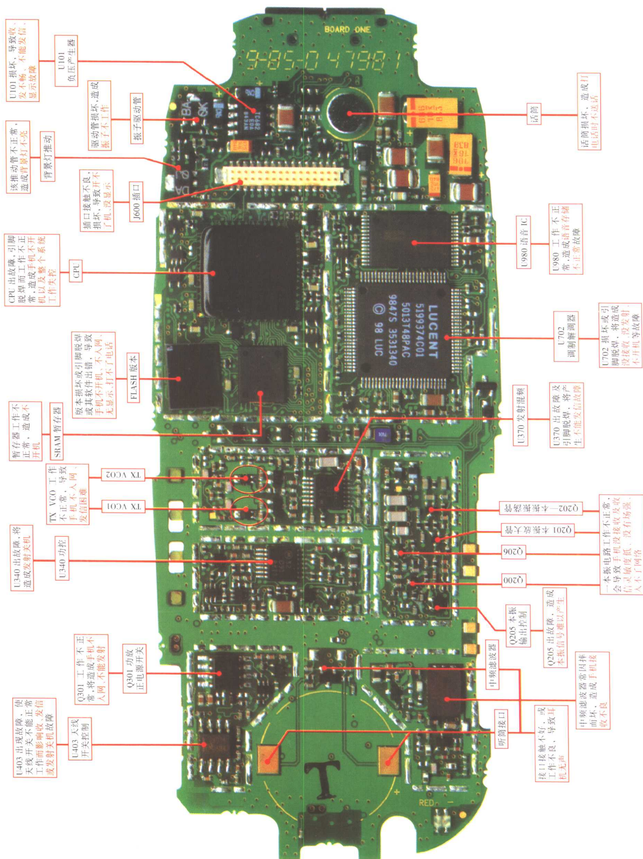
摩托罗拉 cd928 双频手机故障维修彩图(二)
