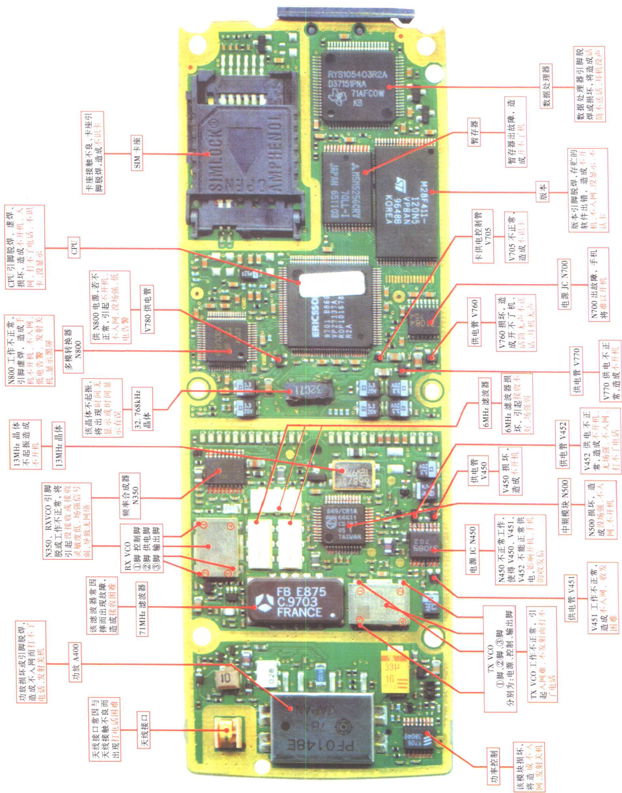
爱立信 388(398)手机故障维修彩图(一)
