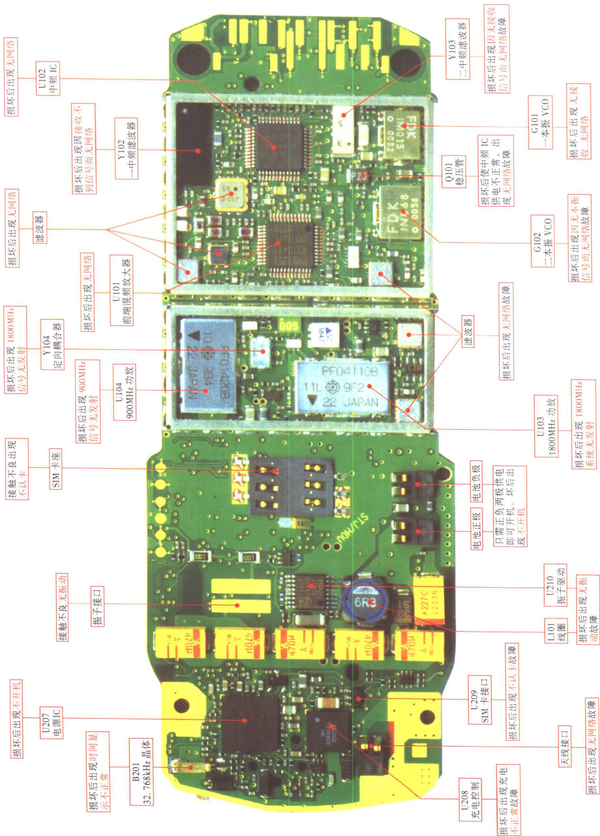
诺基亚 3210 双频手机故障维修彩图(一)
