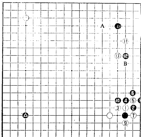
参考谱 1
