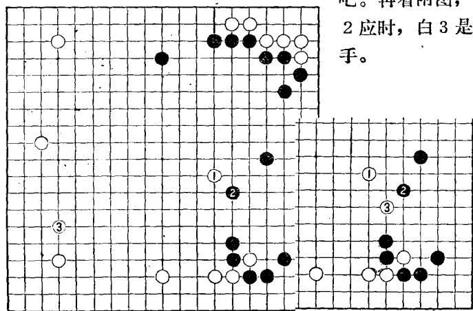
参考谱4
