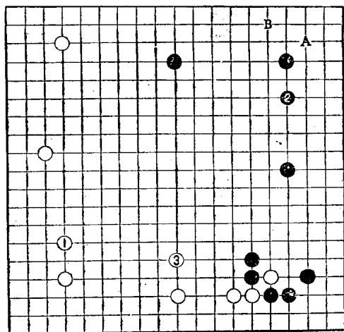
参考谱3
