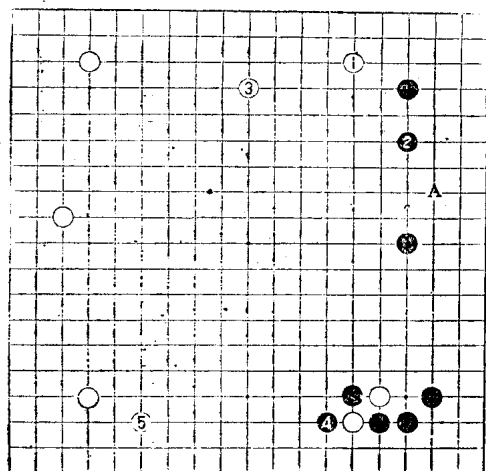
参考谱 2
