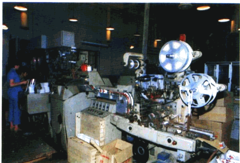
3、西昌卷烟厂新组装的生产线正进行生产。
