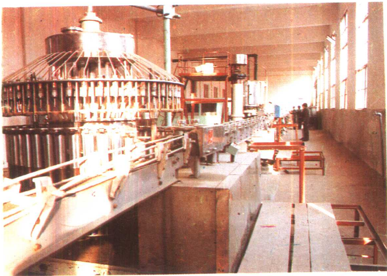
果酒厂白酒生产线
