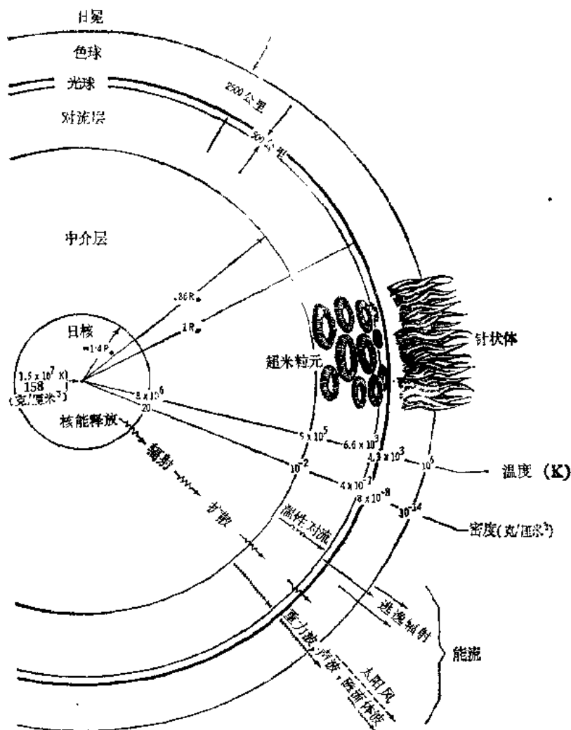
图1-1 太阳总体结构示意图
