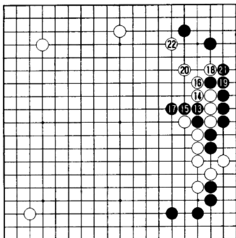
参考谱 2
