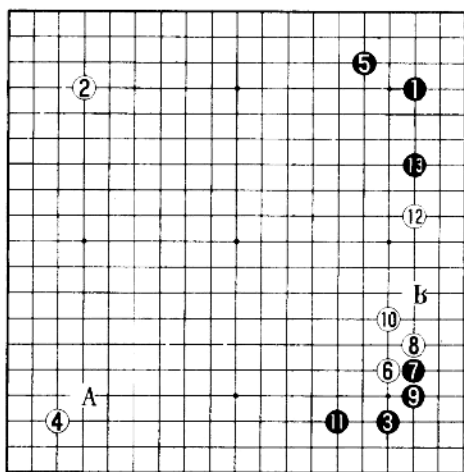
谱 1(1~13)
