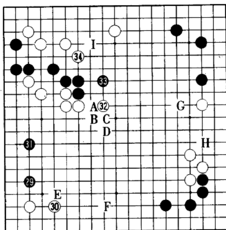
谱 3(29 ~ 34)
