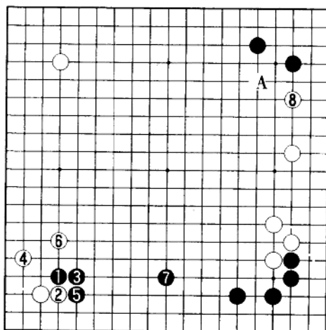
参考谱 1
