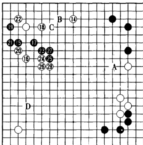
谱 2(14~28)
