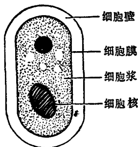
图 I 1-2 细菌细胞基本构造(模式图)
