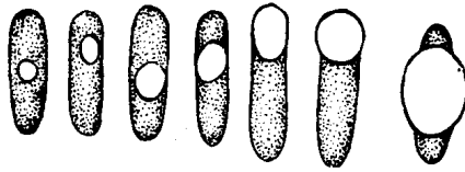
图 I 1-4 细菌芽胞的形态及位置
