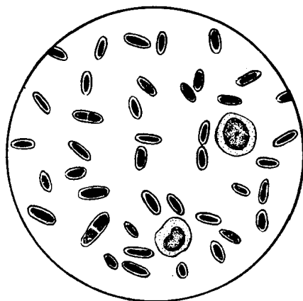
图 I 1-3 细菌的荚膜
