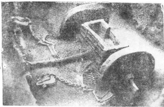
图六 商代车马遗存 河南安阳大司空村出土
