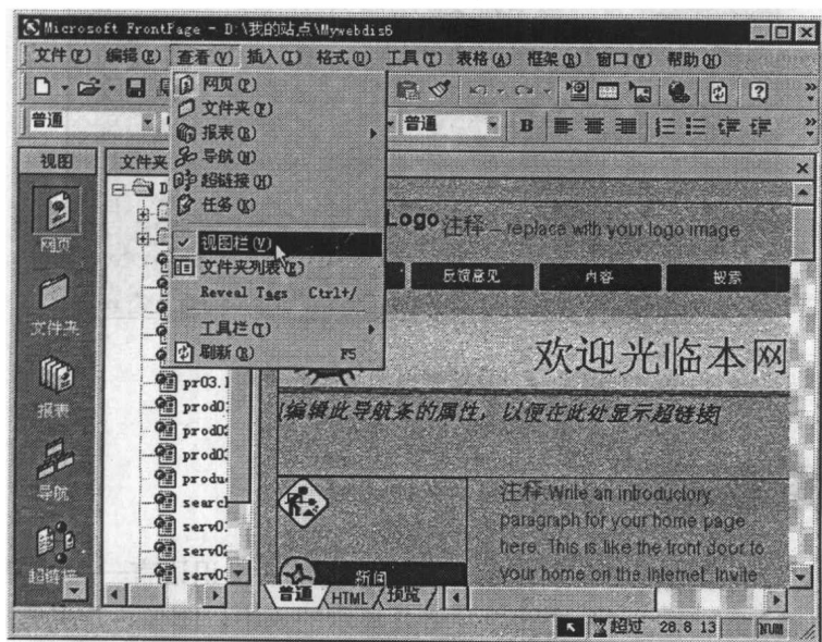
图 1-11 隐藏“视图”栏
