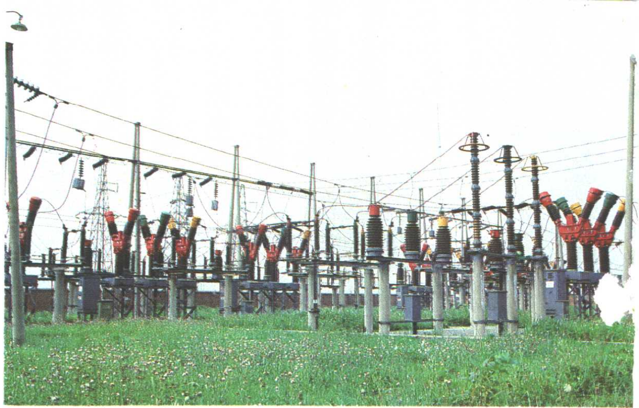
二〇千伏安油坊 变电站
