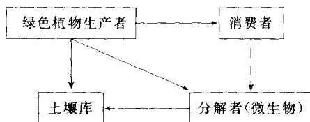
图 1-1 自然生态系统中的物质循环
