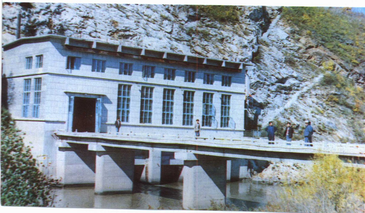
宽河水电站的发电厂房与尾水交通桥
