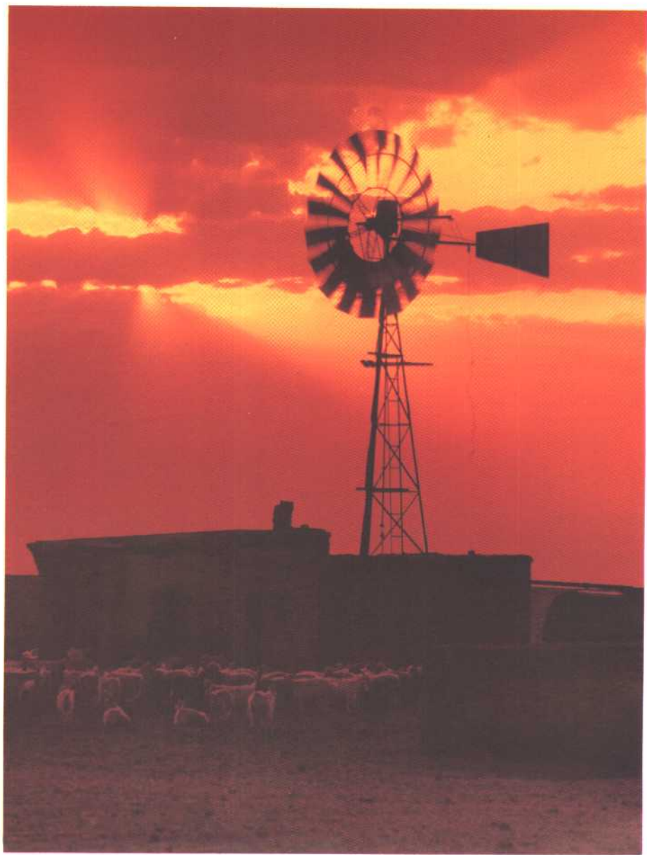
内蒙古巴盟牧区风力提水
