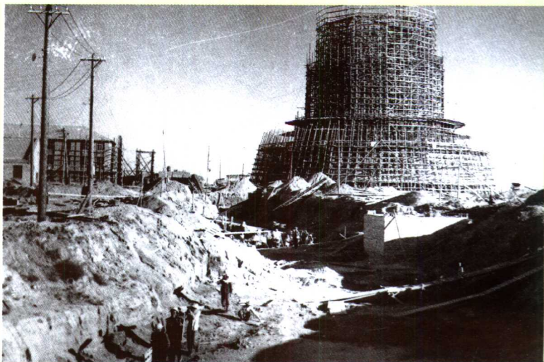
1958年包头第一热电厂在建设
