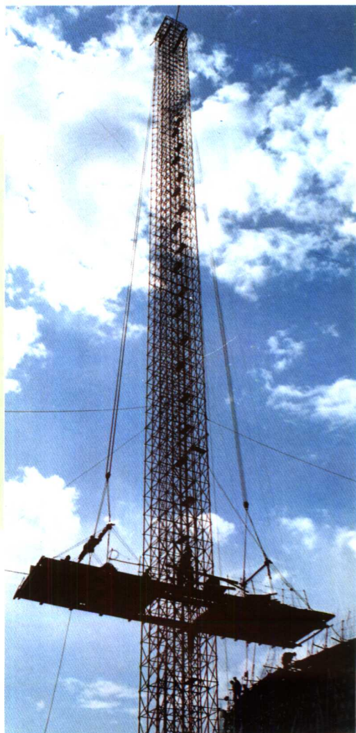
耸立青天——80年代施工机具 (一电厂扩建现场)
