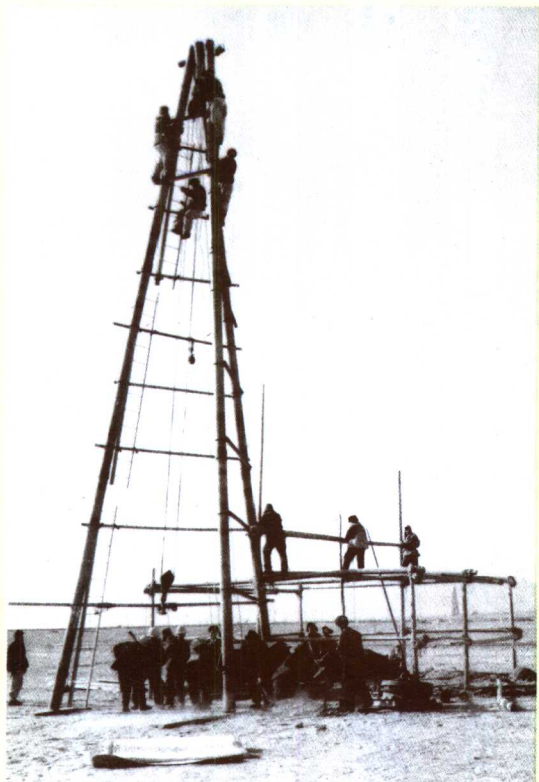
立起木架滑轮——50年代施工机具
