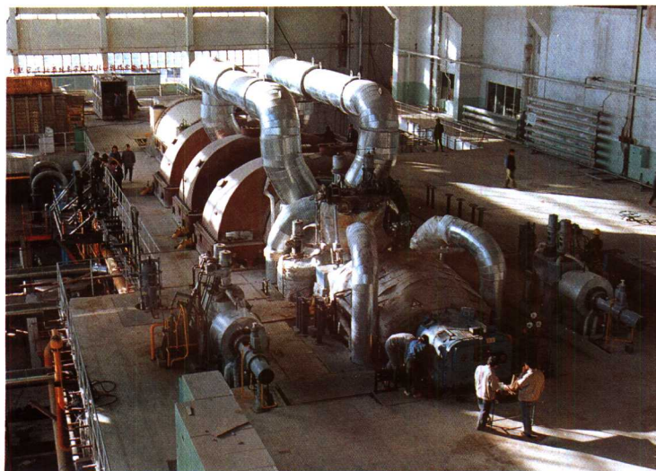
丰镇发电厂第一台20万千瓦机组
