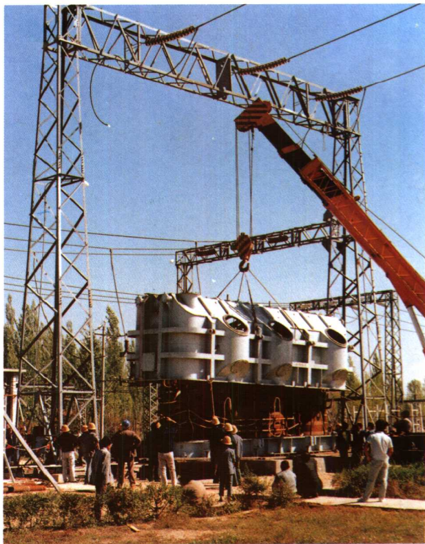
变电站主变在安装
