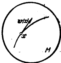
图7 相速度向量.
