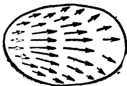
图 8 向量场.
