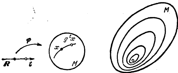
图 4 在相空间 M 中相点的运动。
