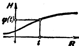
图 6 扩张相空间中的积分曲线。
