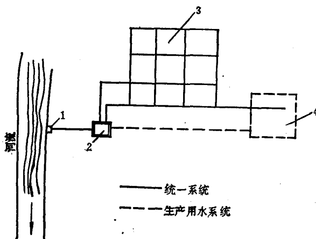
图 1-2 分质给水系统
