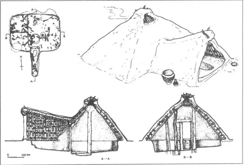
西安半坡FH复原图
