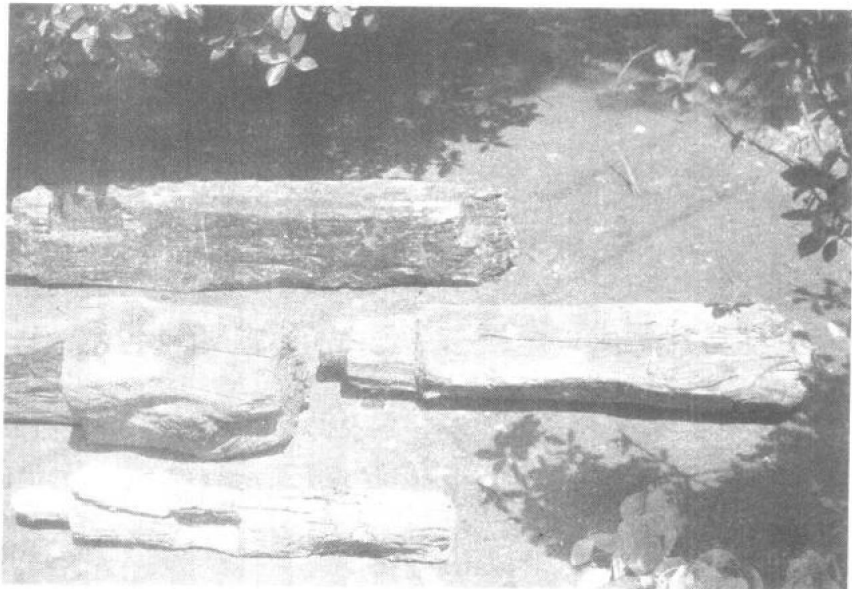
浙江余姚河姆渡出土的榫卯构件实物图
