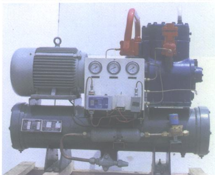
蒙城安徽省冷冻机厂所产的部优产品 2F6.5 制冷压缩机
