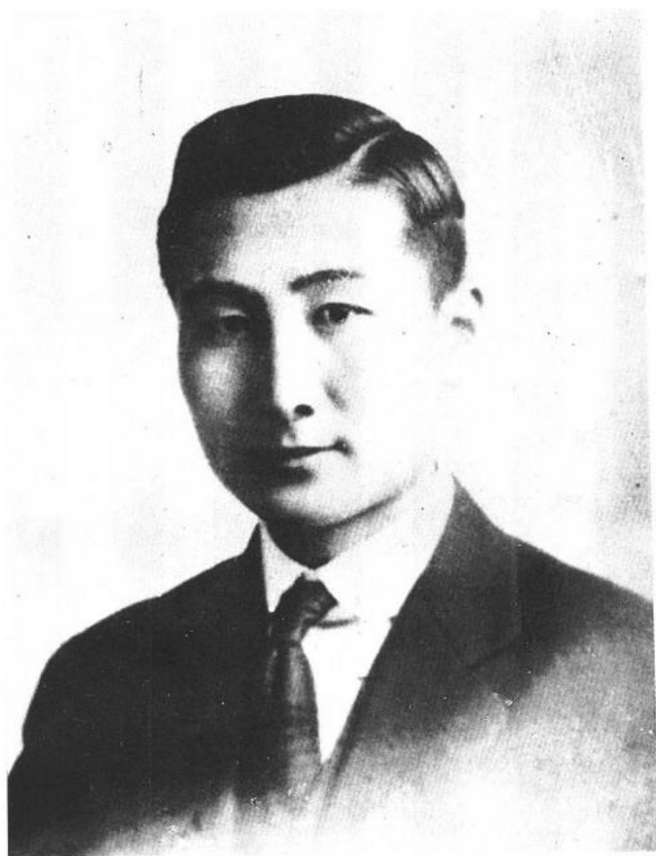
王希天烈士
