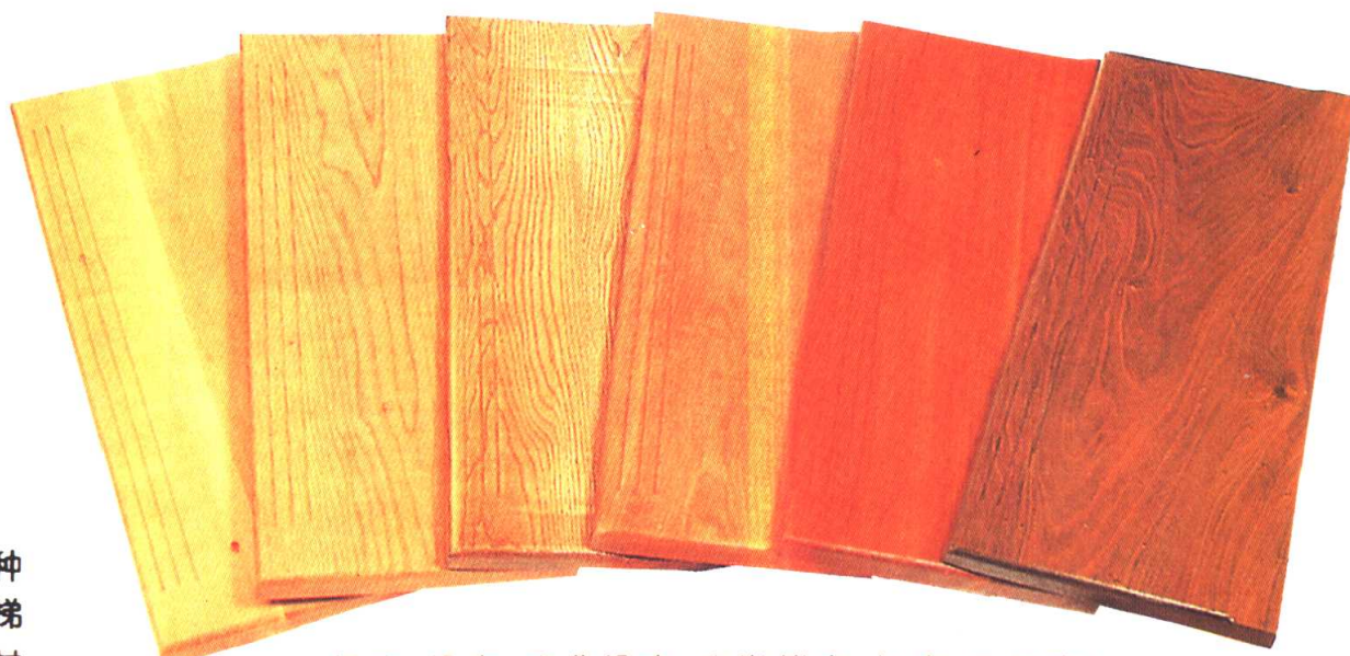
常用的企口型木地板
