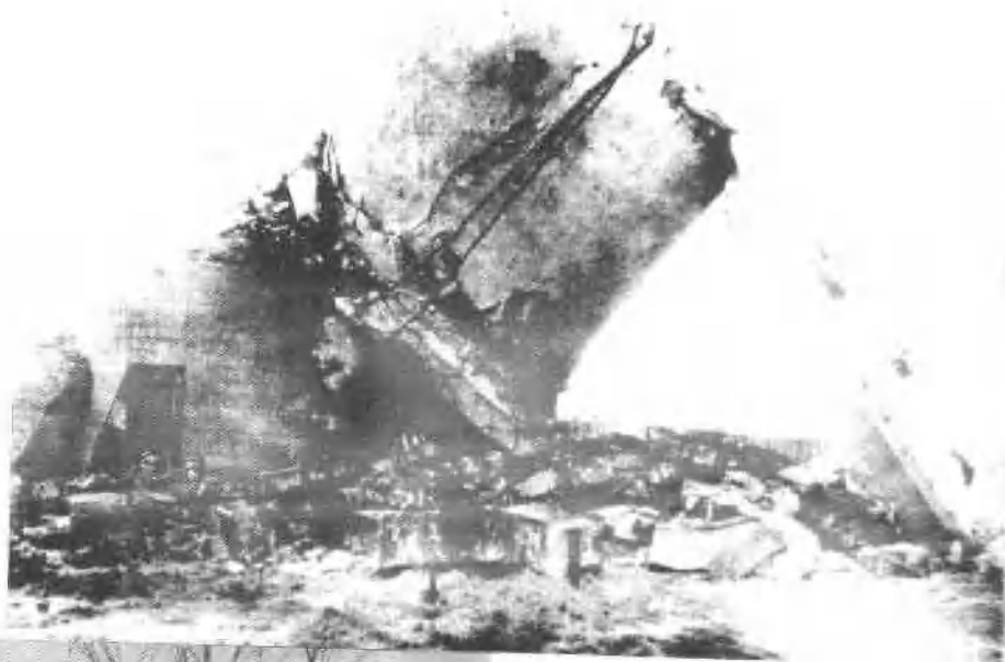
2. 汉沽天津旭日化工厂,高26米的水塔,底座为砖结构,储水池为钢筋混凝土结构,震后座塌池坠。
