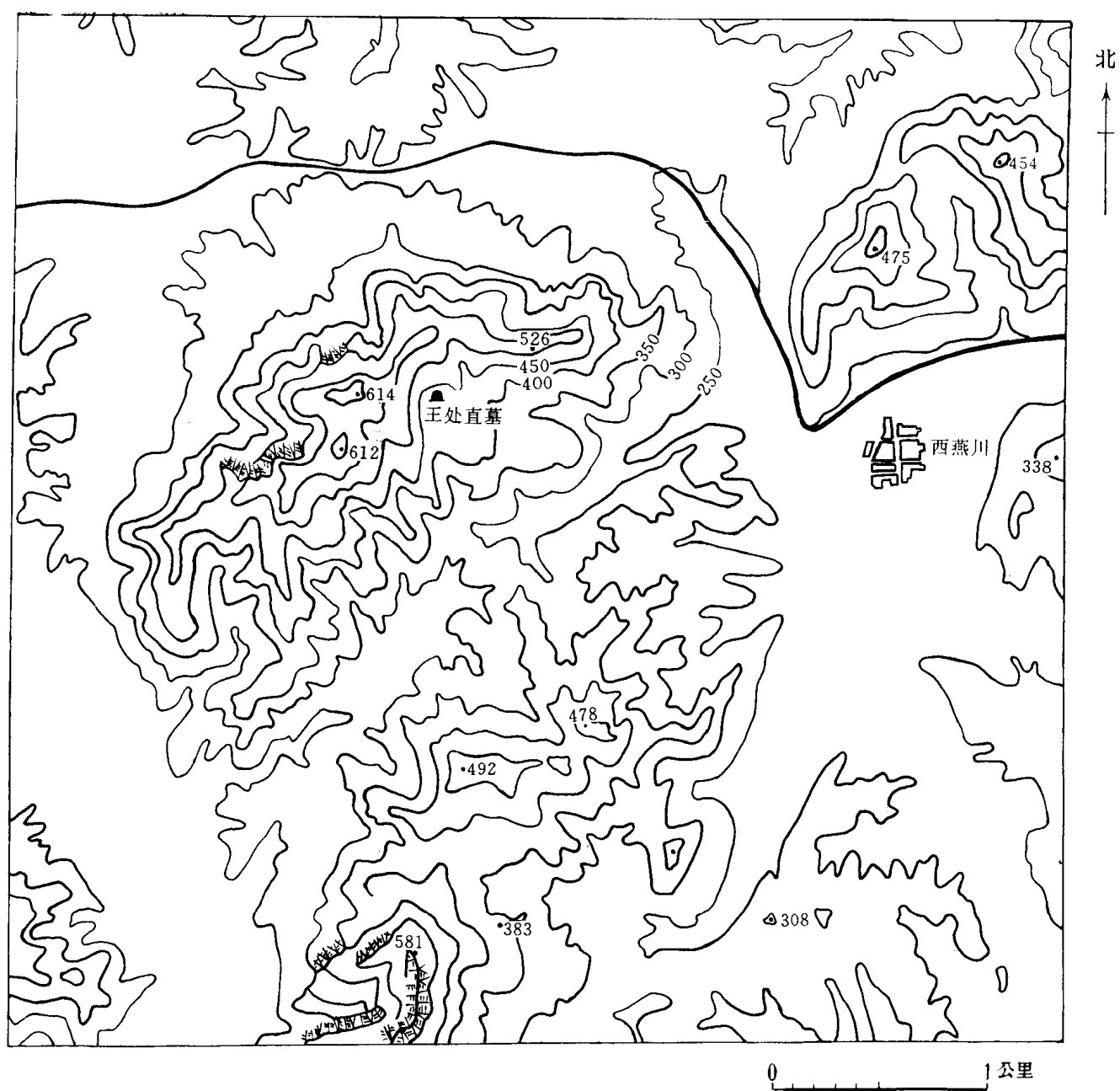
图二 墓葬周围地形图
