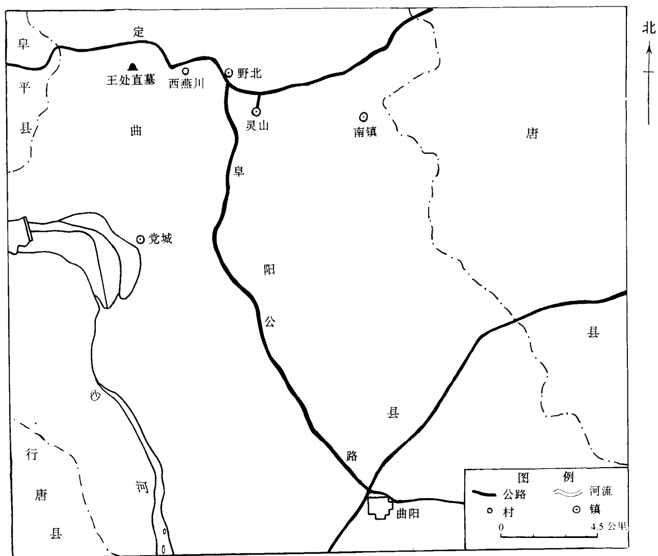
图一 墓葬地理位置图
