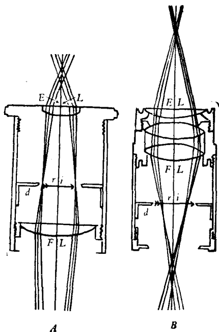
图 1-3 图示惠更斯目镜(A)及补偿目镜(B)
