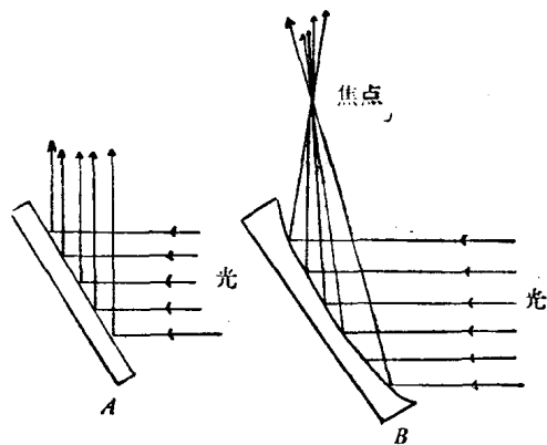
图 1-4 反光镜的反光样式
