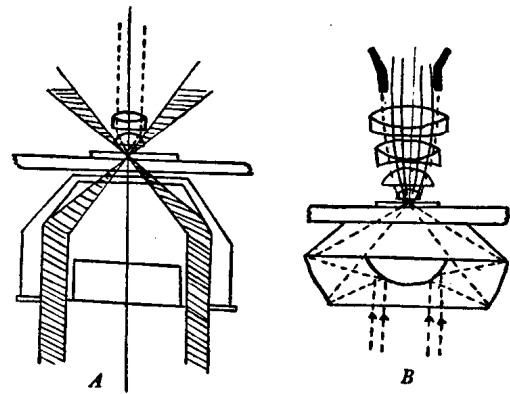
图 1-5 暗视野聚光镜
