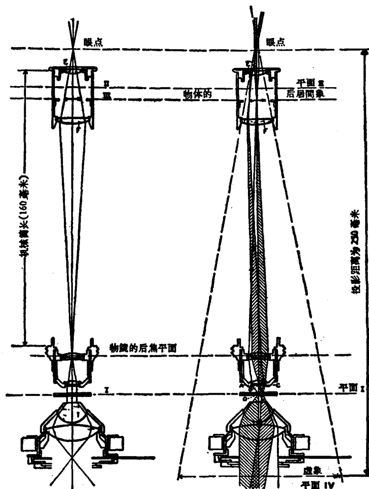
图 1-2 光线通过显微镜时的途径
