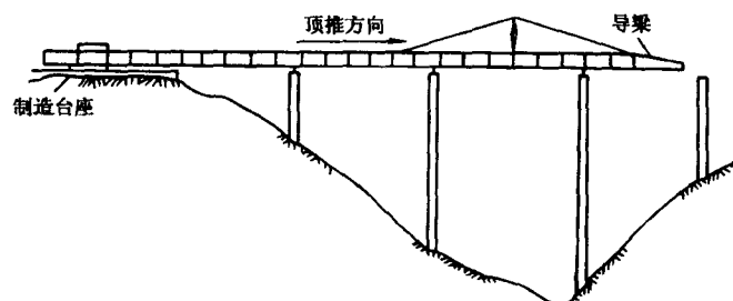
图 2-1 顶推法施工示意
