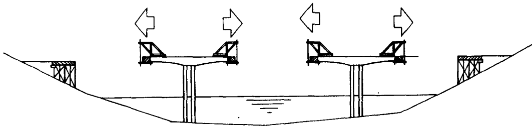
图 2-2 混凝土梁桥悬臂施工示意
