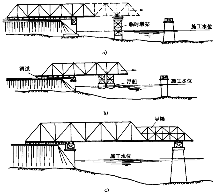
图 2-3 钢梁桥拖拉施工示意
