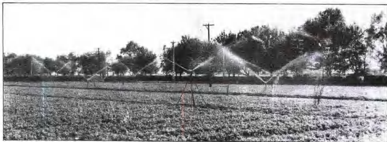
长春市二道河子区英俊乡福利村露地蔬菜生产喷灌实况
