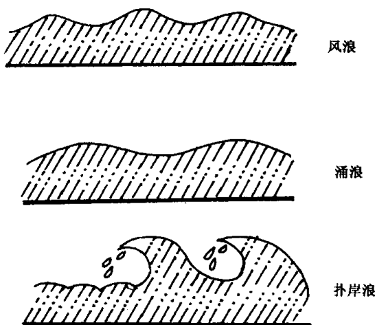
图 1.1 风浪、涌浪、扑岸浪
