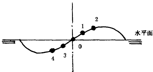
图 1.2 水分子的运动
