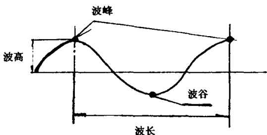
图 1.3 波浪的构成
