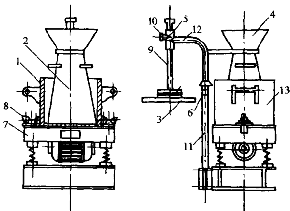
图 1-2 维勃稠度仪
