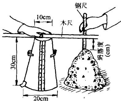
图 1-1 混凝土拌合物 坍落度值的测定
