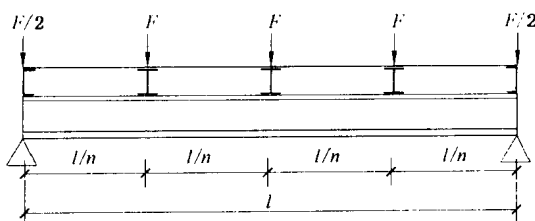
图 2-6 简支梁的间接荷载
