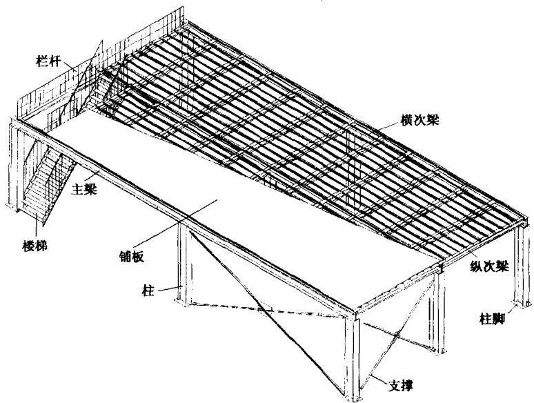
图 2-1 平台结构布置
