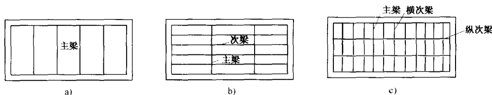
图 2-2 梁格布置
