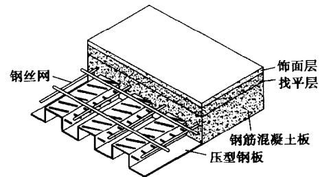
图 2-5 压型钢板与钢筋混凝土的组合楼板
