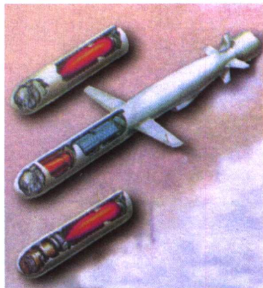
“战斧”的三种型号解剖图。
