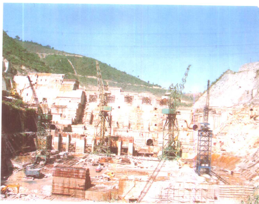
漫湾电站大坝工地
